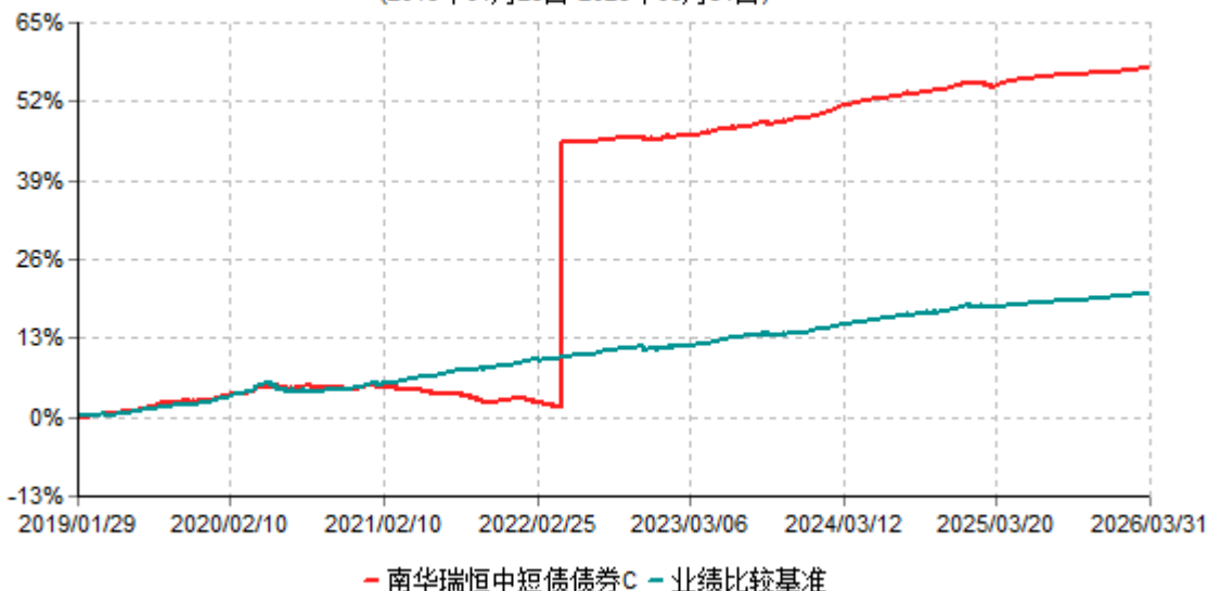
南华瑞恒中短债债券C累计净值增长率与业绩比较基准收益率历史走势对比图 (2019年01月29日-2026年03月31日)
